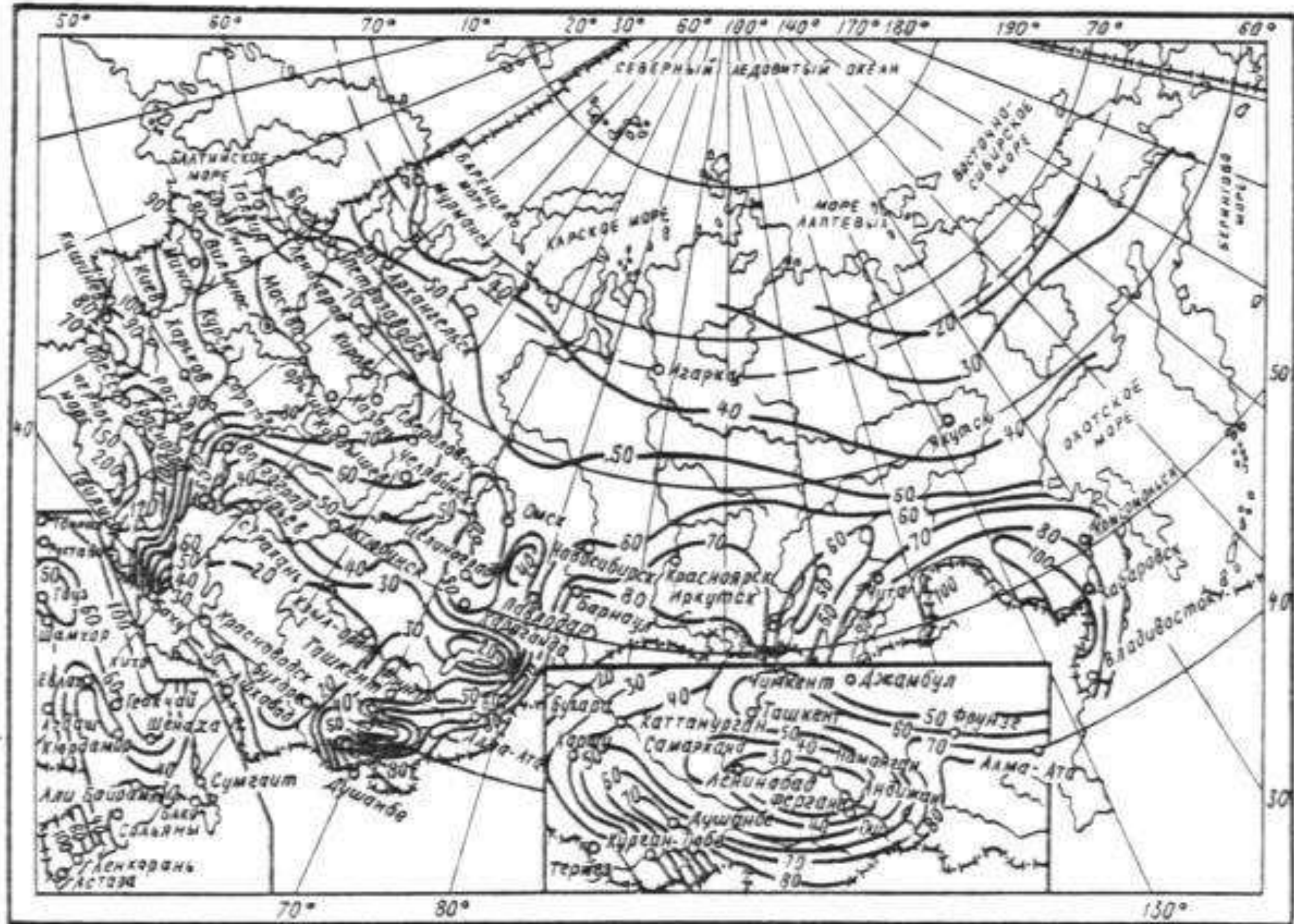
Черт. 1. Значения величин интенсивности дождя q_{20}
