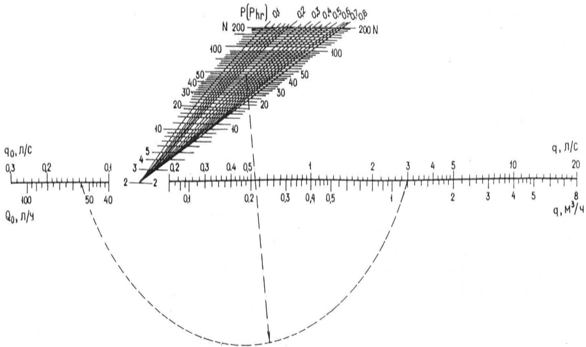
Черт. 3. Номограмма для определения секундных и часовых расходов воды q при q_0 \leq 0,3 л/с, N \leq 200 и P > 0,1
